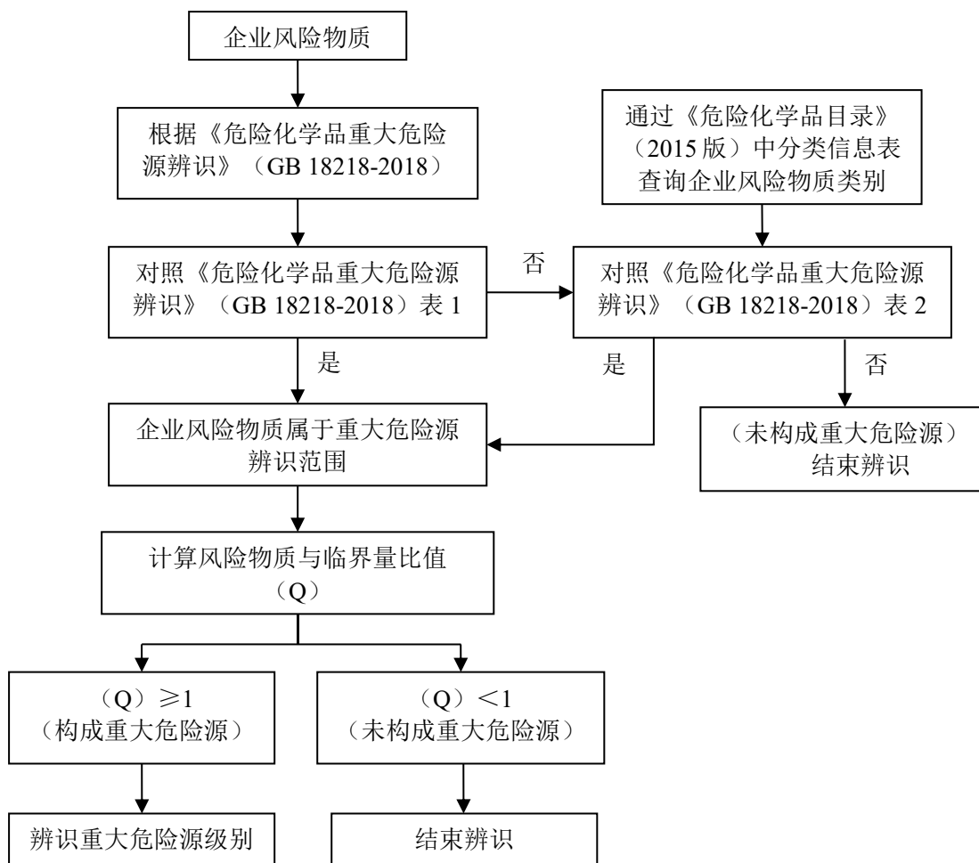
3.4-1 企业重大危险源辨识流程图
