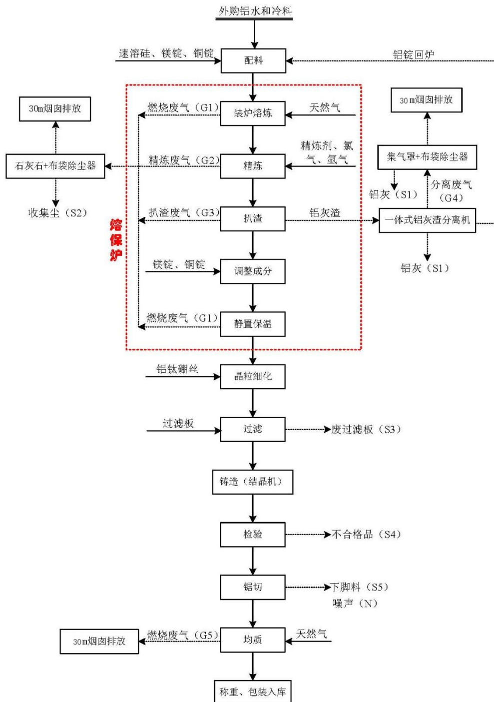
4.2-1 项目 120 万吨/年生产工艺流程图
